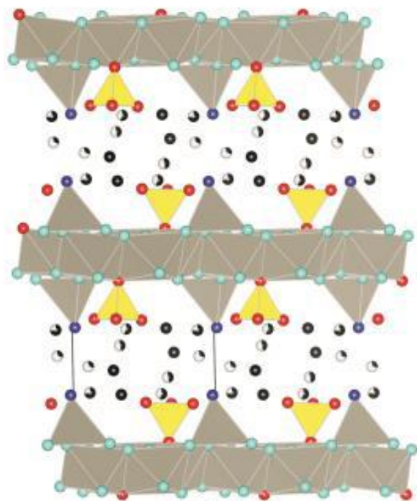
osakaite \text{Zn}_4(\text{OH})_6\text{SO}_4 \cdot 5\text{H}_2\text{O}
